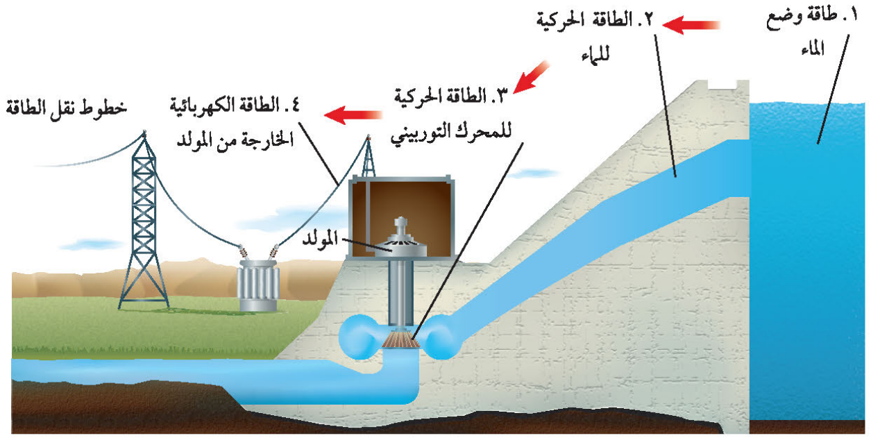
الشكل ٥ طاقة الوضع خلف السد تزود التوربين بالطاقة لتشغيله. فسر. لماذا تُعد الطاقة الكهرومائية مصدرًا متجددًا للطاقة؟
