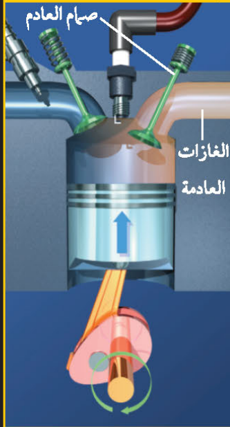
شوط العادم
