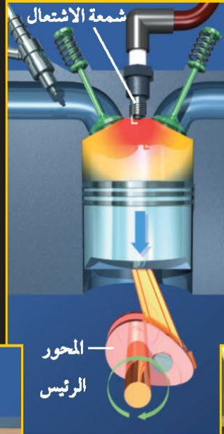
شوط الاشتعال
